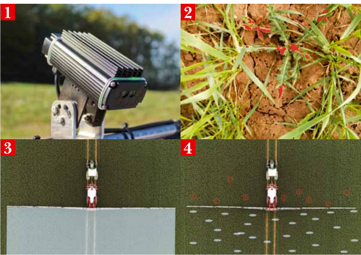
1 Vysokospektrálny senzor na detekciu burín s LED prísvecovaním pri zlých svetelných podmienkach.; 2 Detekcia nežiaducich burín.; 3 Systém I-SPRAY je deaktivovaný, postrekovač strieka celoplošne podľa nastavenej dávky; 4 Postrekovač s aktívnym systémom I-SPRAY, pri ktorom vysokospektrálne senzory snímajú zaburinenosť porastu a následne aplikujú herbicíd pomocou jednotlivých trysiek samostatne. Týmto systémom je možné ušetriť až 90 % nákladov na postrek.
